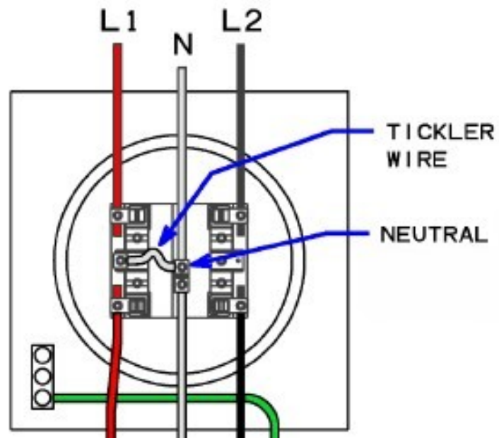
5 JAW METER SOCKET
